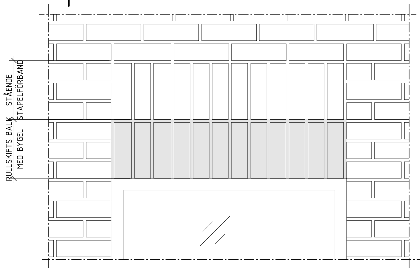
EV1 PRINCIP ELEVATION
