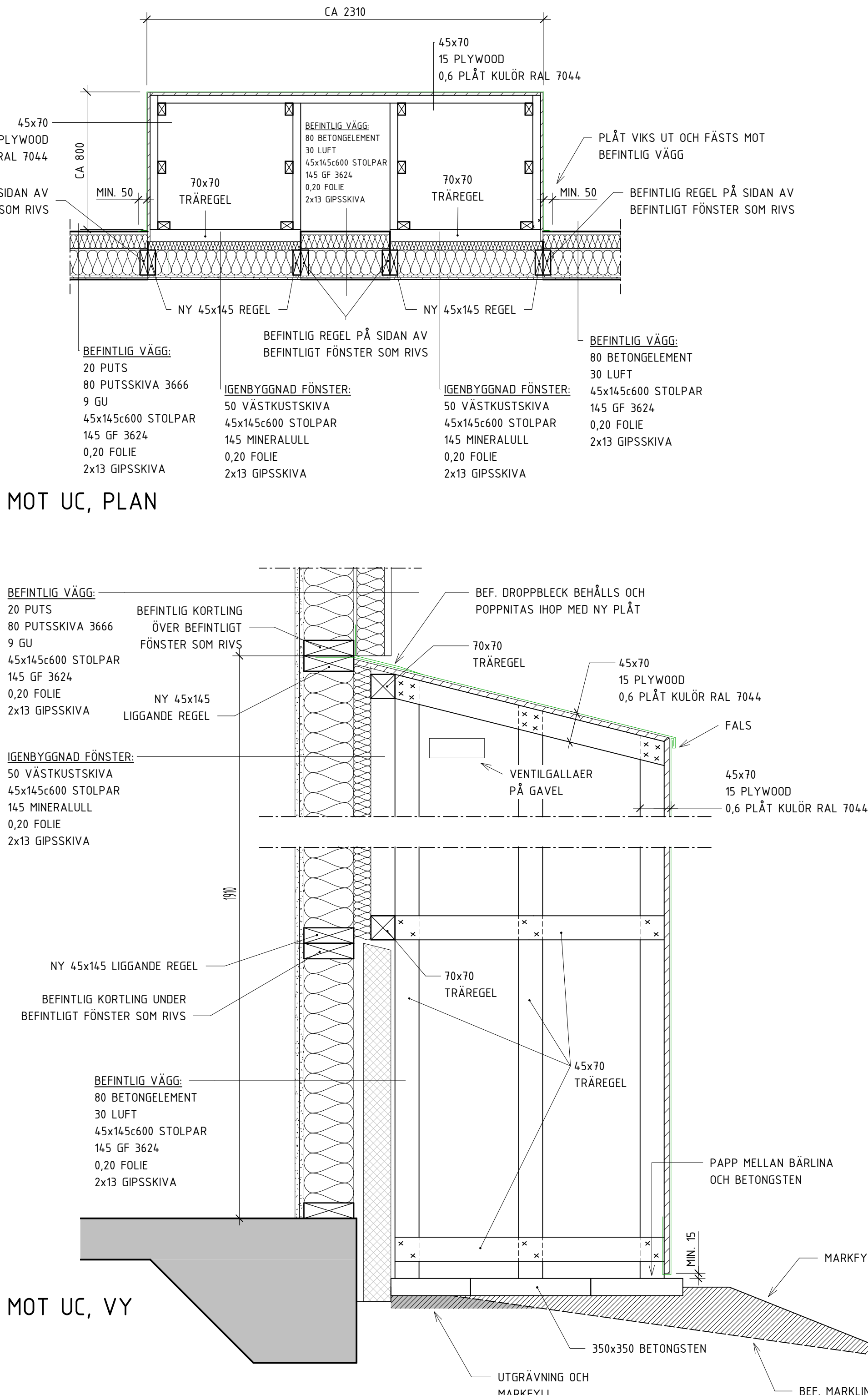
EV2 PRINCIP ELEVATION
