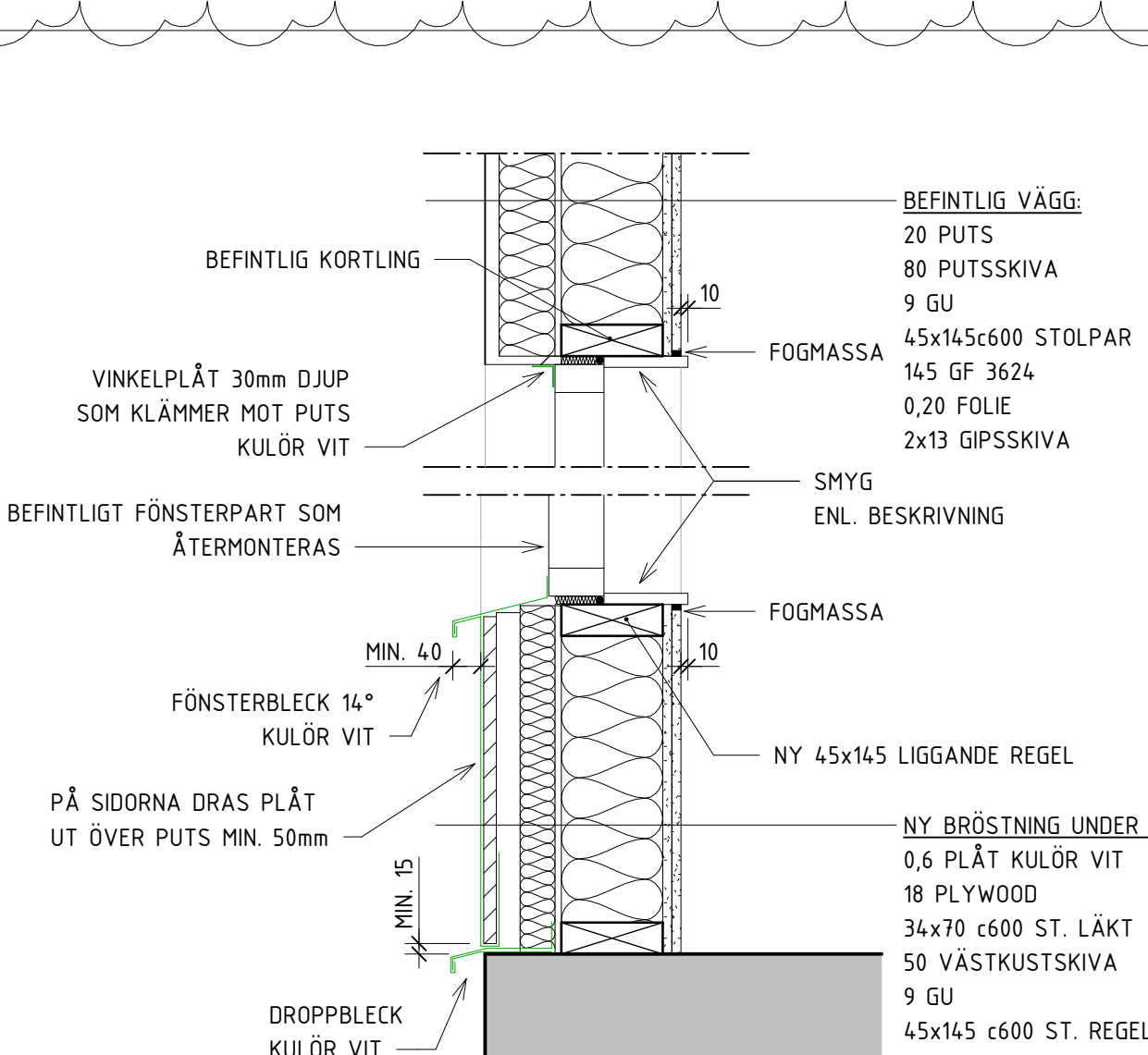
VD22 - IGENBYGGNAD FÖNSTER FRITIDS
